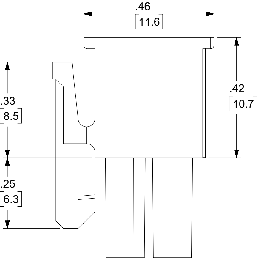
4 CKT SHOWN
